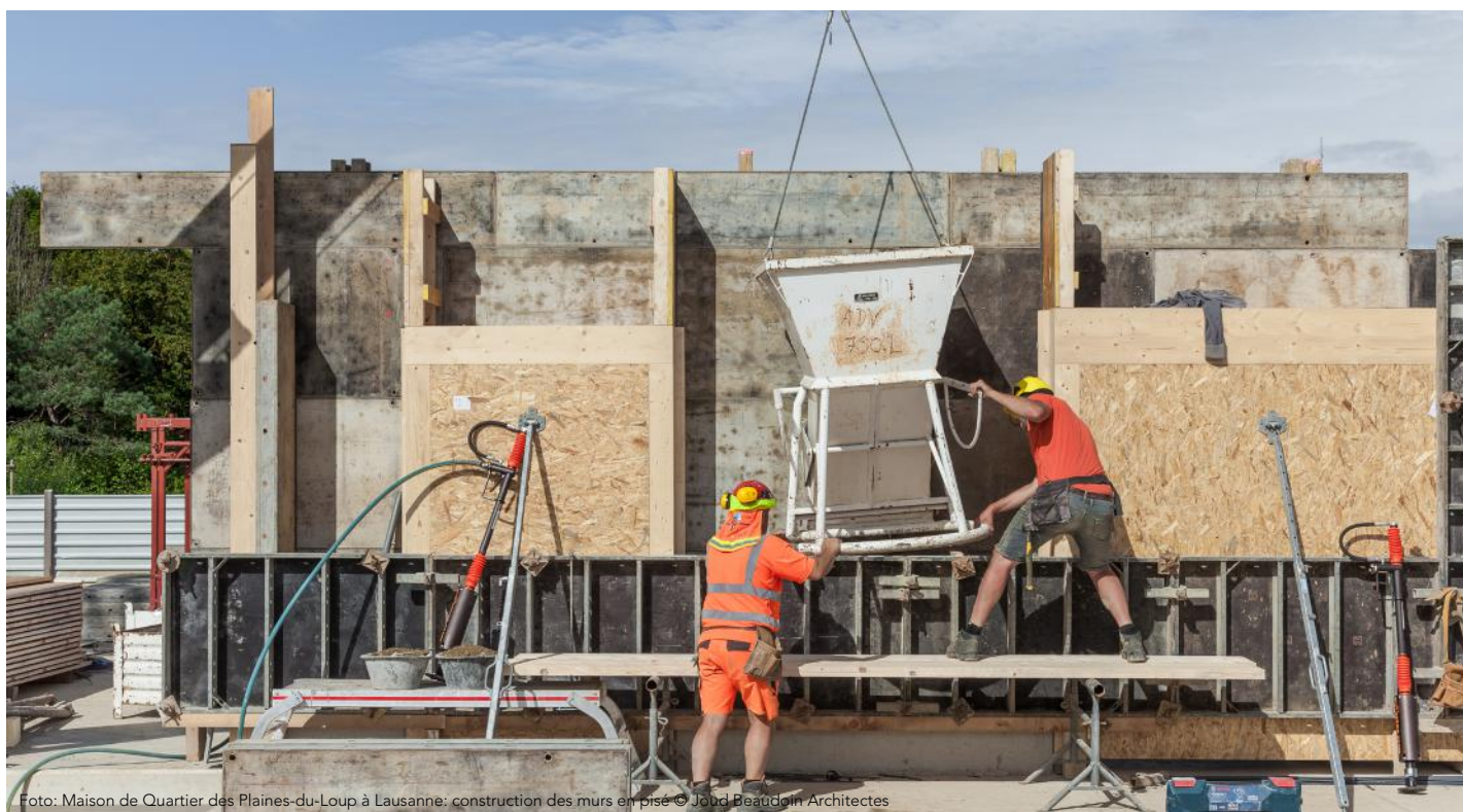
Foto: Maison de Quartier des Plaines-du-Loup à Lausanne: construction des murs en pisé © Jodé Beaudoin Architectes
