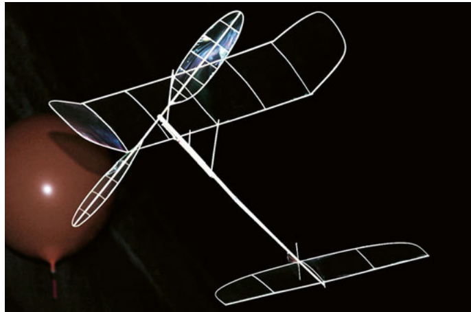
Indoor-Modelle Klasse F1D-Saalflug werden mit Ballons gesteuert.
